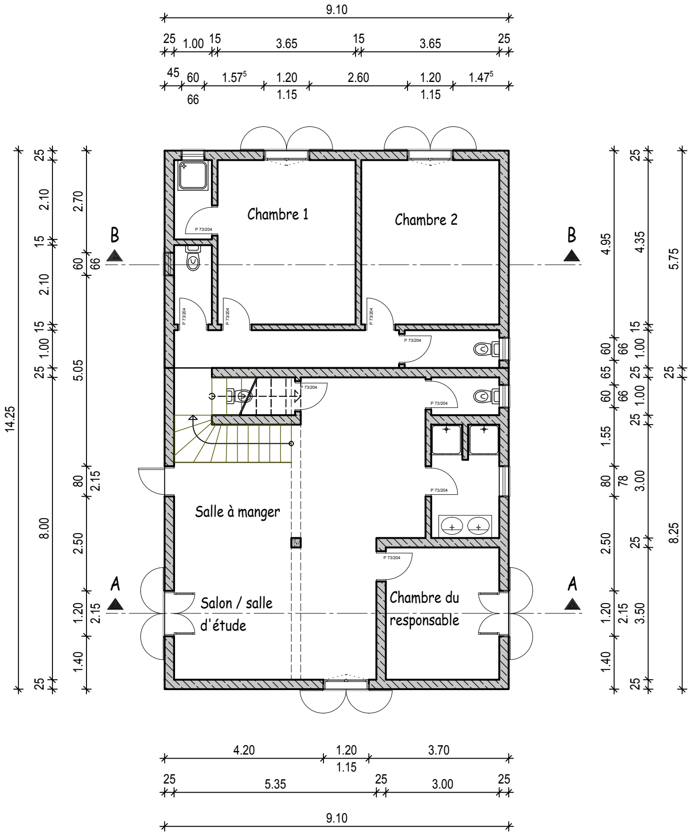
VUE PLAN RDC
