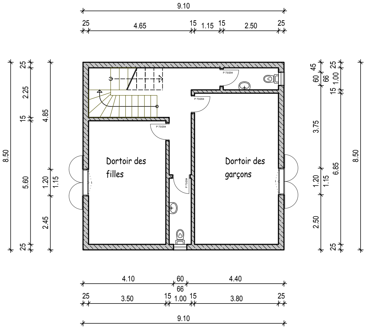
VUE PLAN ETAGE
