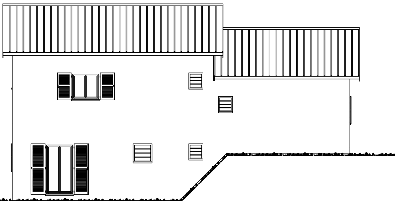
FACADE LATERALE DROITE
