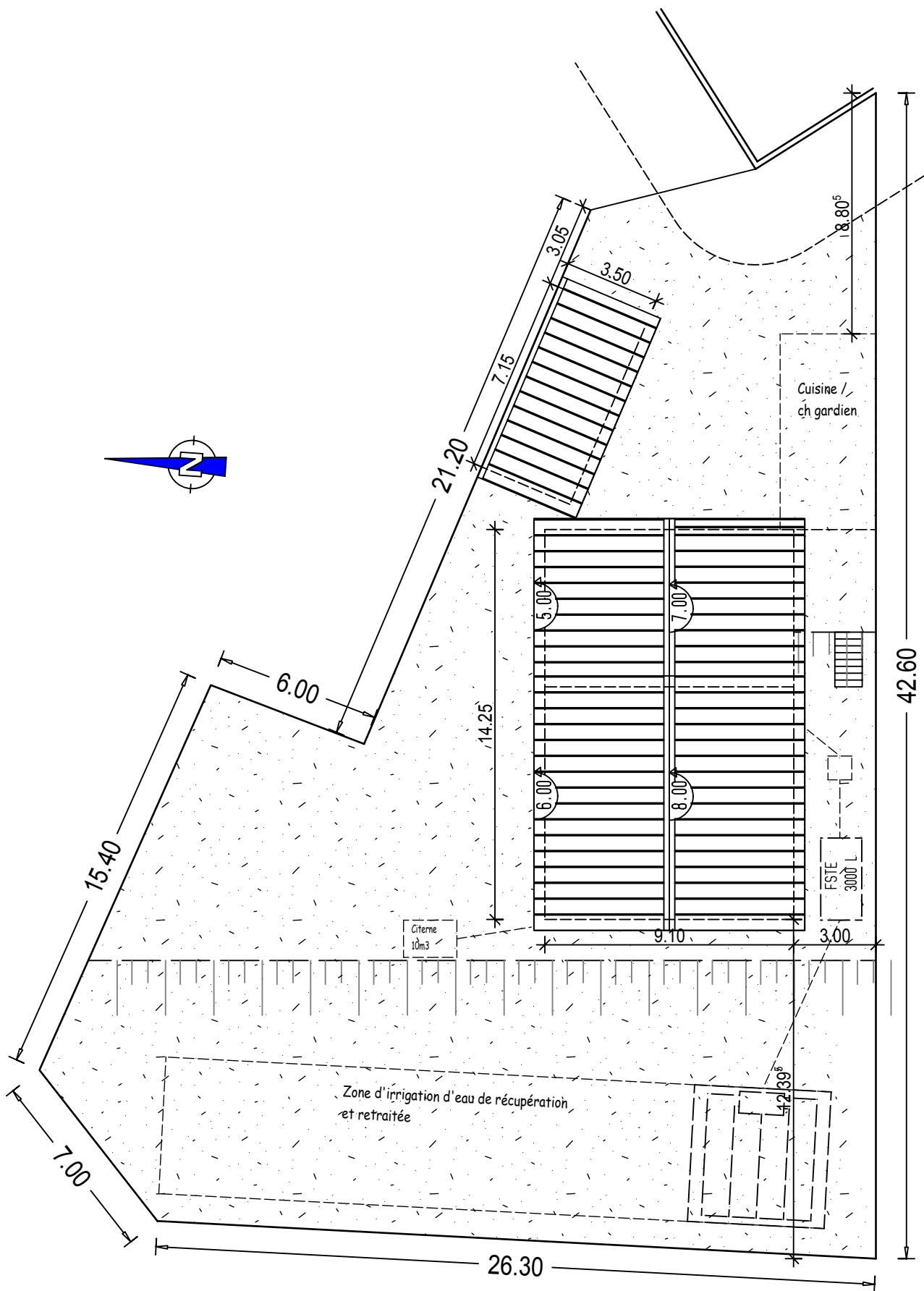
PLAN D'IMPLANTATION Echelle : 1/200
